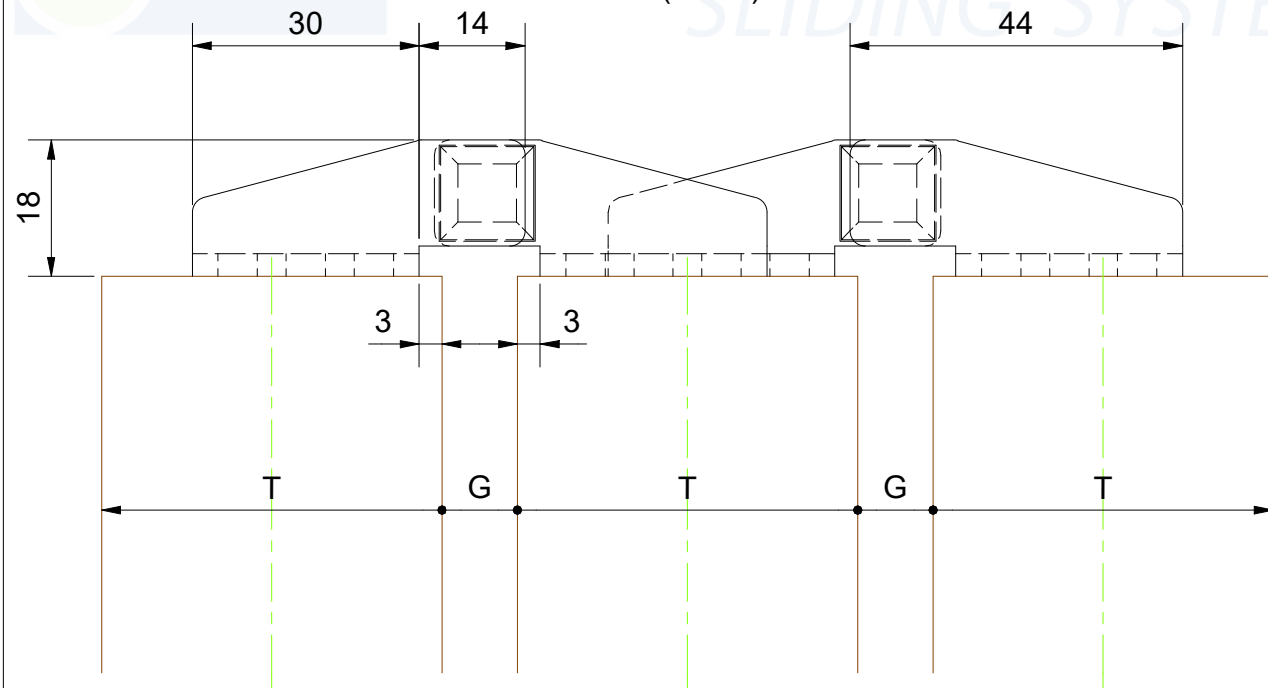
C-C (1 : 1)
