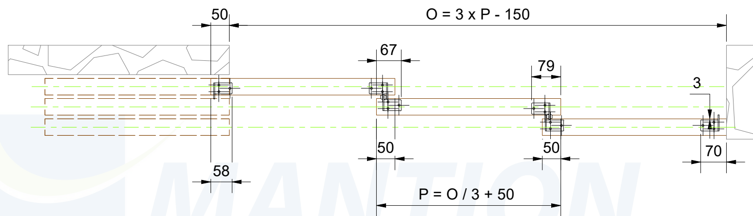
B-B (1 : 10)
