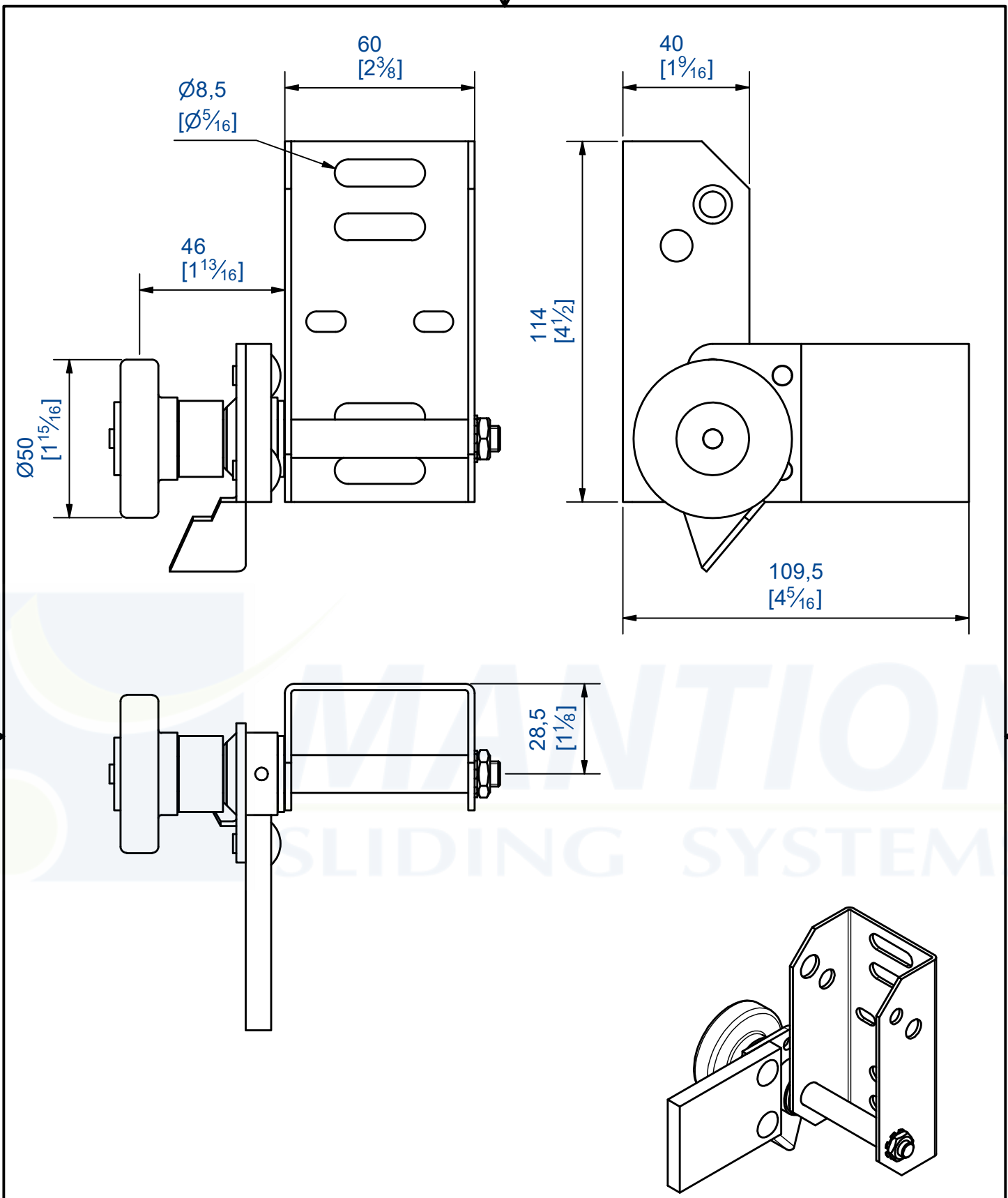
Guide gauche avec galets acier et parachute de sécurité
