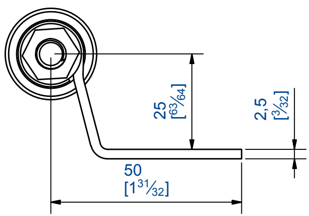
Guide du bas d'extrémité déporté pour U 30x30. (1110) Offset bottom guide for u-profile 30x30 (1110).
