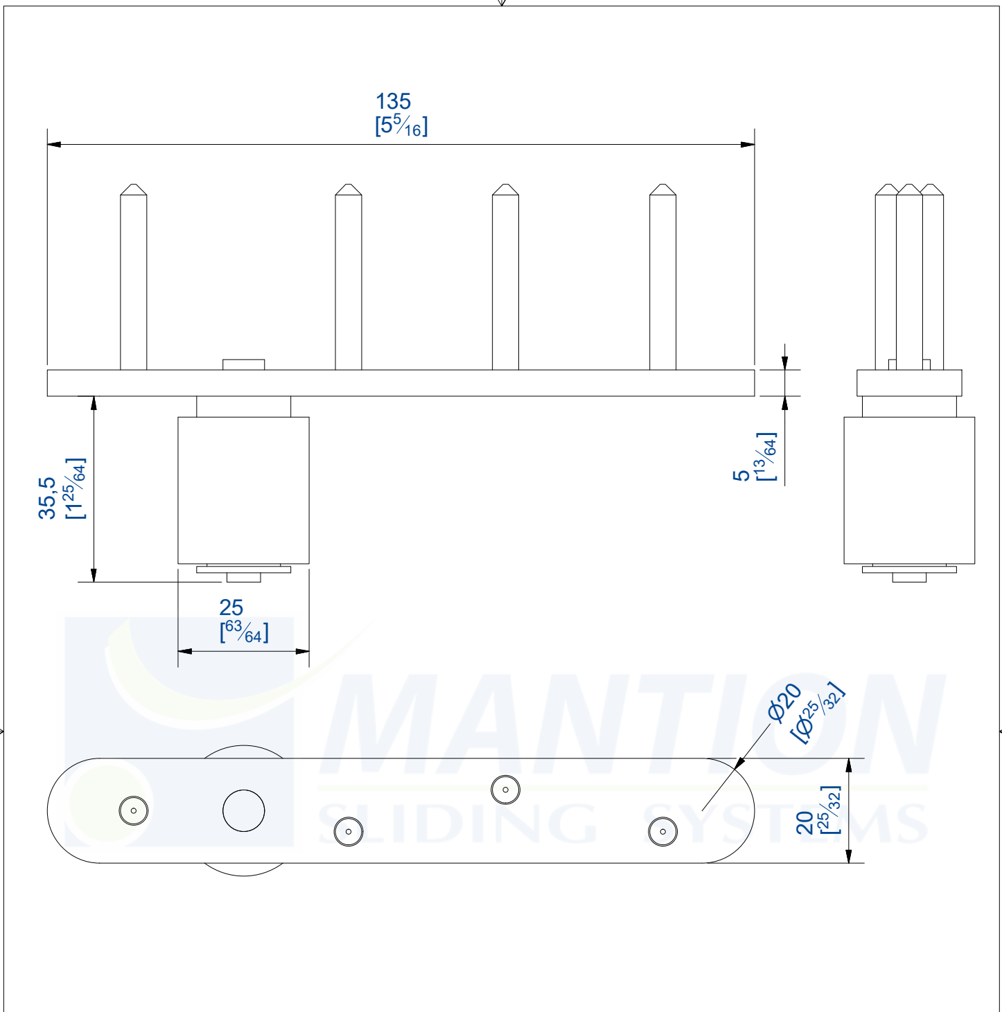
GUIDE BAS SUR PLATINE A VISSER POUR 1110 BOTTOM GUIDE ON PLATE FOR U30X30
