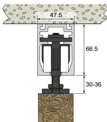
Houten deurmontage 13044
