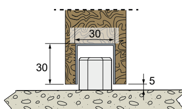
Bodenführung 1110GDL + Profil 1110
