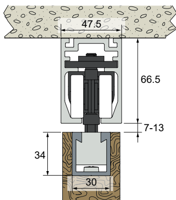
Holzmontage mit Platte 13040 + Profil 28FC
