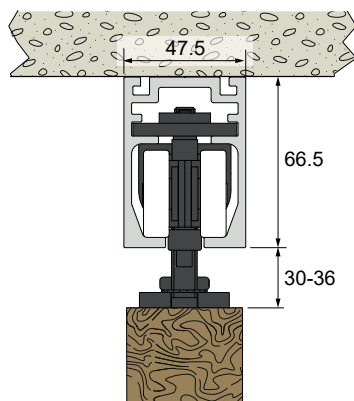
Holzmontage mit Platte 13044
