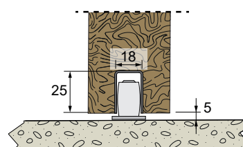
Bodenführung 1102 + Profil 1109A
