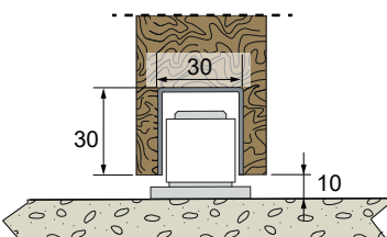
Guide 1081 + profile 1110
