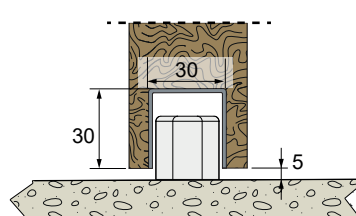
Guide 1110GDL + profile 1110
