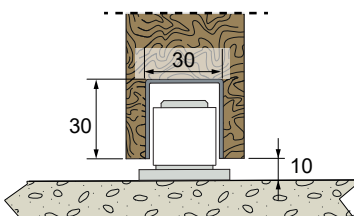
Bodenführung 1081 + Profil 1110
