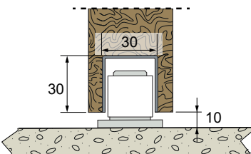
Bodenführung 1081 + Profil 1110
