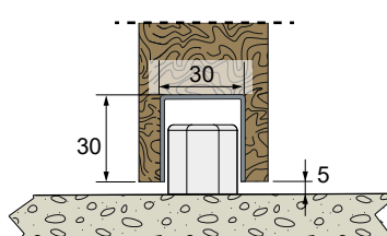
Bodenführung 1110GDL + Profil 1110
