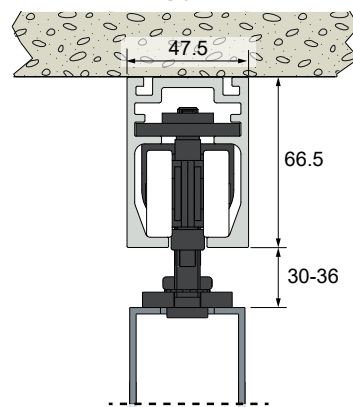
Metallmontage mit Platte 13044
