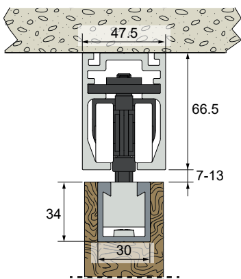
Holzmontage mit Platte 13040 + Profil 28FC
