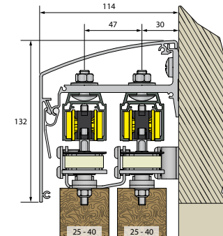
Muurbevestiging tweewegs gesynchroniseerd
