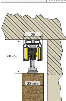
Plafondbevestiging
