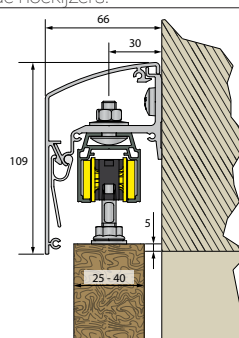
Muurbevestiging eenwegs
