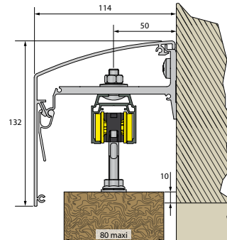
Muurbevestiging (zonnescerm)
