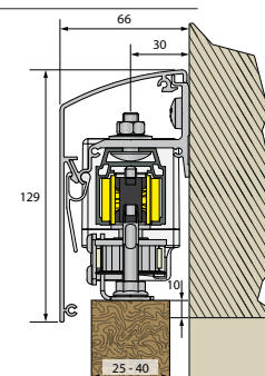
Muurbevestiging eenwegs gemotoriseerd
