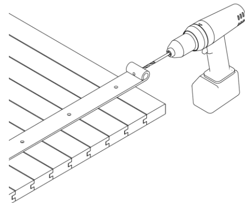
Perçage parallèle
