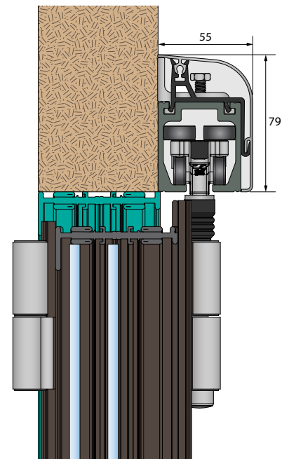
Coupe partie haute
