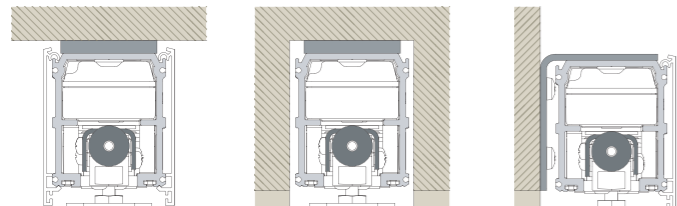
DECKENBEFESTIGUNG
