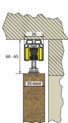
Fixation plafond 1 voie - manuel
