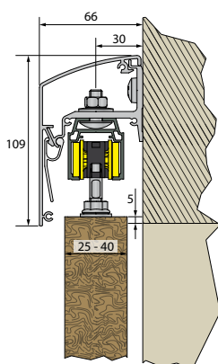
Fixation murale 1 voie - manuel
