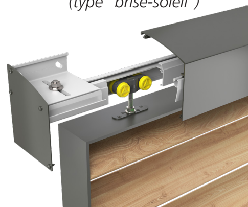
Fixation murale 1 voie - manuel (type "brise-soleil")
