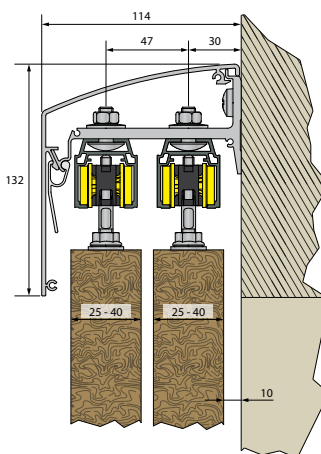
Fixation murale 2 voies - manuel
