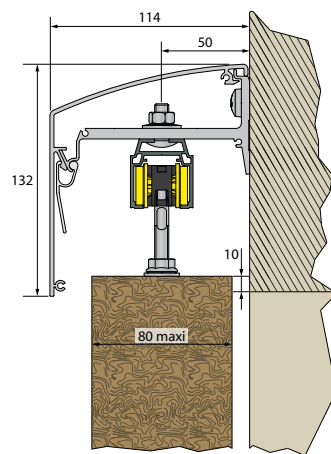
Fixation murale 1 voie - manuel (type "brise-soleil")
