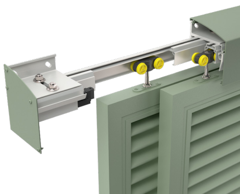
Fixation murale 1 voie - manuel
