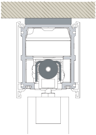
DECKENBEFESTIGUNG
