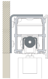
WANDBEFESTIGUNG
