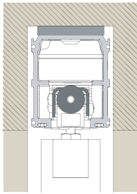
EINGELASSEN
