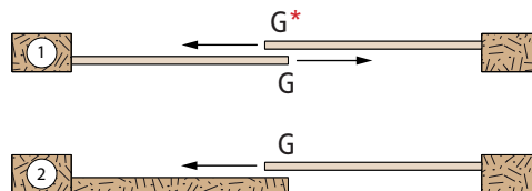
G* : guide bas 1123
