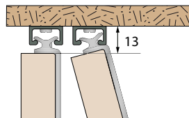
Patin 0111 démontable
