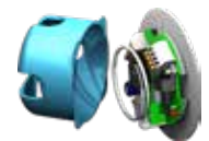
Steuergerät mit versetzt angebrachter Elektronik
