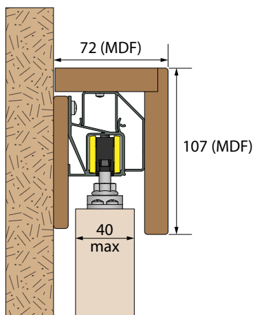
Schnittansicht der Montage
