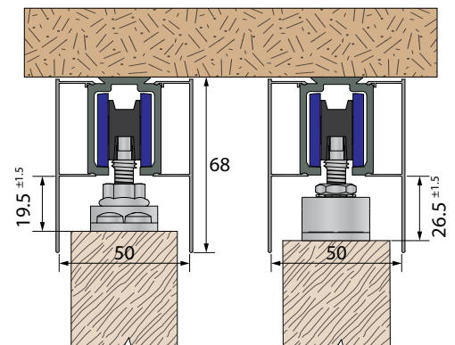
Deckenbefestigung mit Platte 10036 Deckenbefestigung mit Platte 11036
