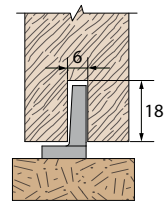
Montage der Führung 1103
