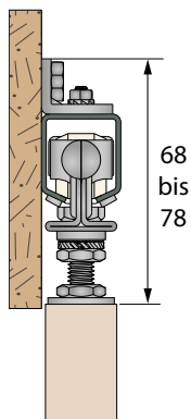
Winkel 2528 für Paneele bis 20 mm Stärke
