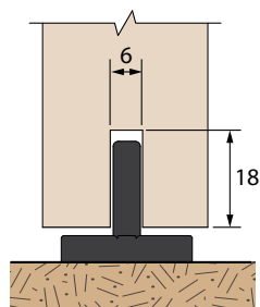
Montage der Führung
