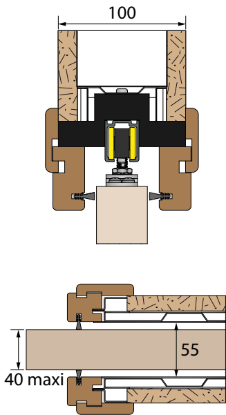
Rahmen-Schnittansicht
