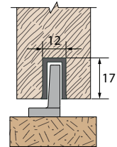
Montage der Führung mit Profil 1106/110
