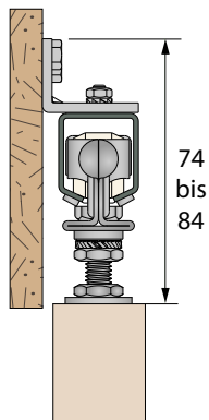
Winkel 2529 für Paneele von 25 bis 40 mm Stärke
