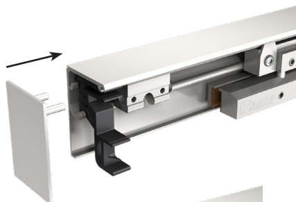
Rail fixation plafond + bandeau
