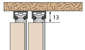
Patin 0112 non démontable
