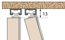
Patin 0111 démontable
