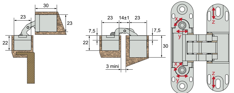
Charnière 1540 encombrement réduit
